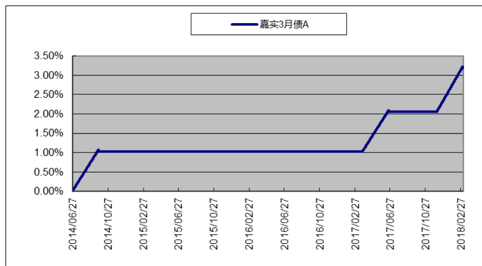
图1: 嘉实3个月理财债券A基金累计净值收益率的历史走势对比图 (2014年6月27日至2018年3月6日)
