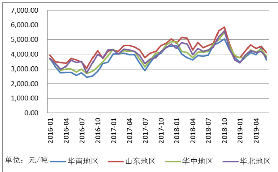
2016 年度至 2019 年 1-6 月国内主要区域 LPG 市场价格走势
