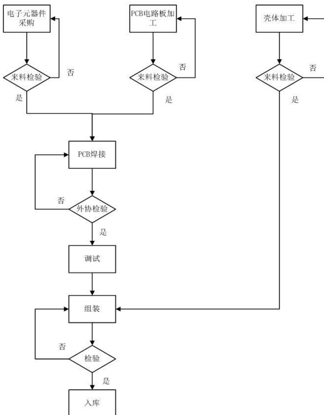
投币机电电子配件生产工艺流程图
