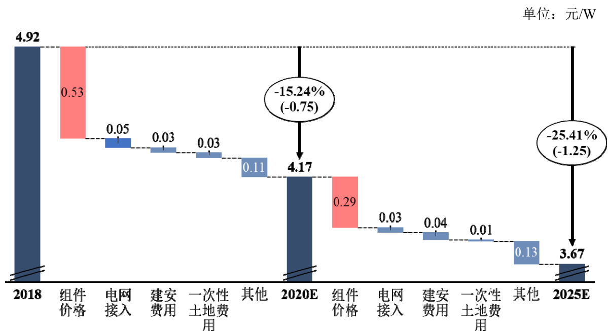
2018-2025 年我国地面光伏系统的初始投资变化趋势
