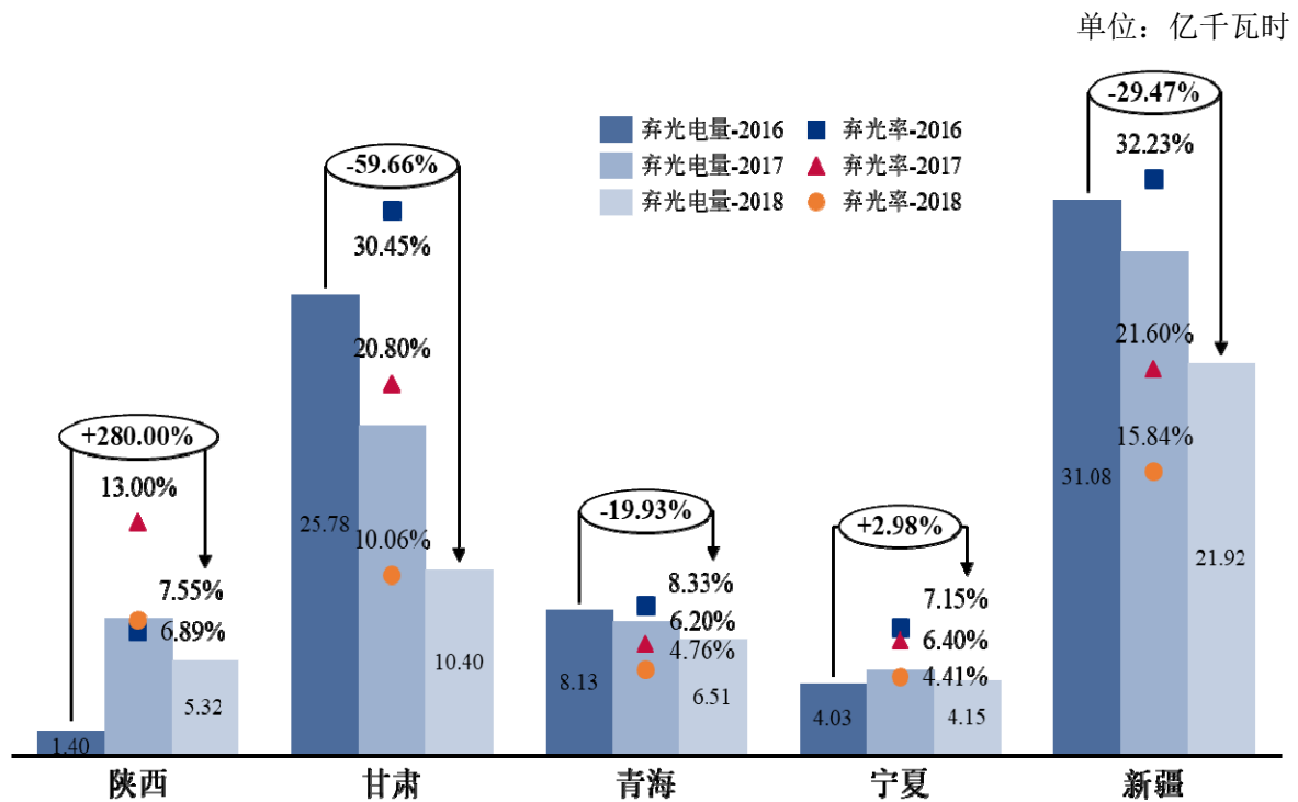
西北地区弃光电量与弃光率
