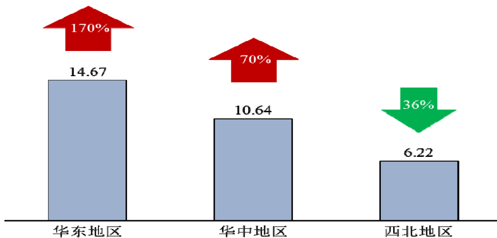
2017 年全国不同地区光伏发电新增装机对比（单位：GW）
