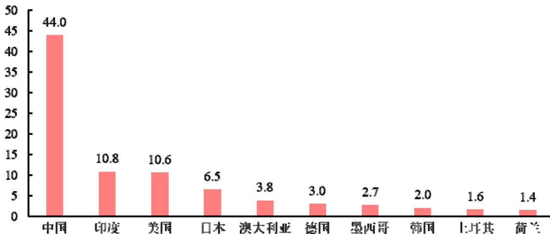
2018 年光伏发电新增装机容量前十大国家
