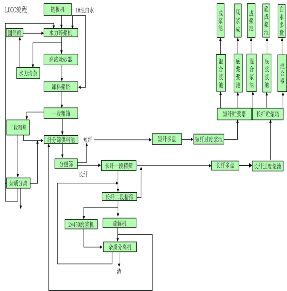
制浆流程
