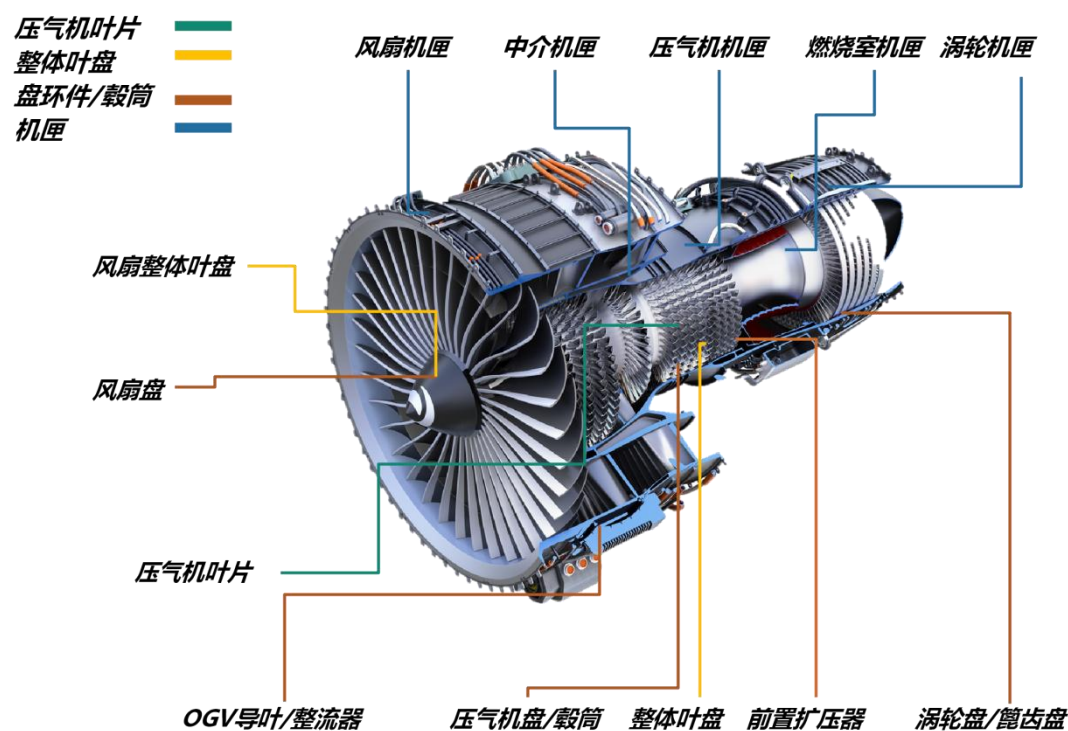
典型航空民用发动机结构示意图
