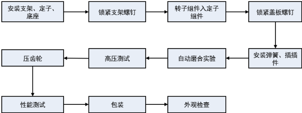
电动工具整机生产工艺流程图（以吹风机为例）
