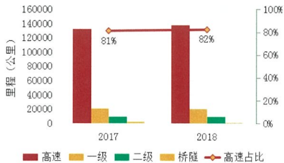
图 1：2017 年~2018 年全国收费公路里程变化图
