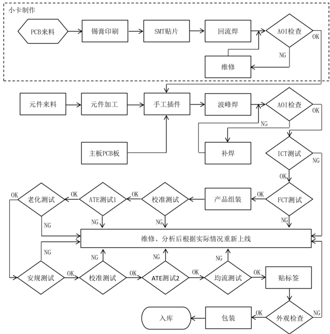
服务器电源主要工艺流程图如下图所示：
