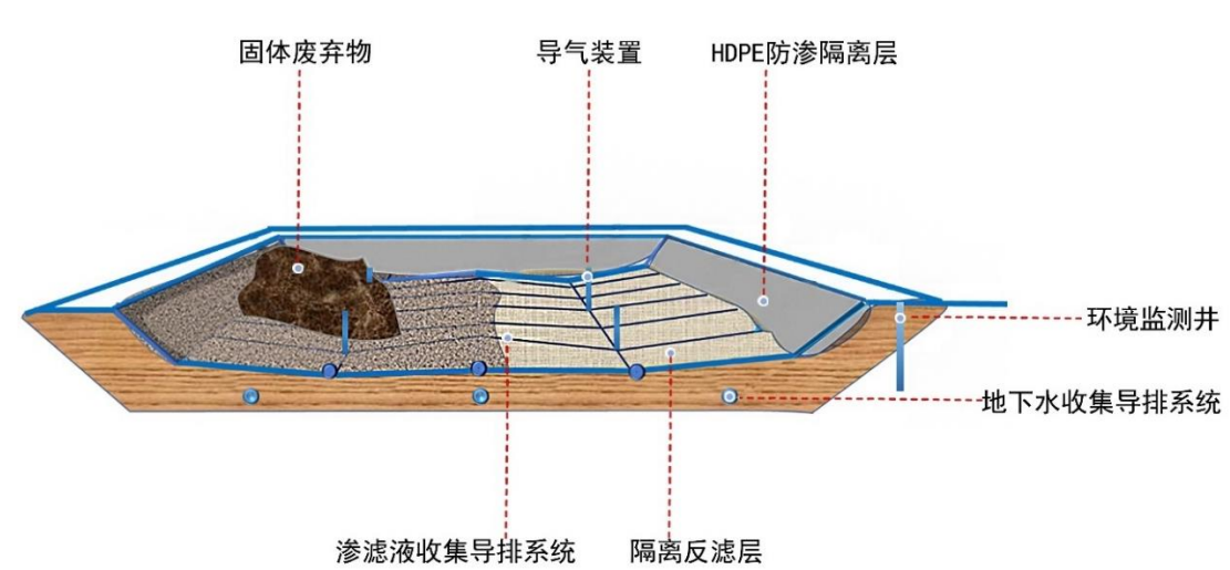
基底防渗隔离系统示意图
