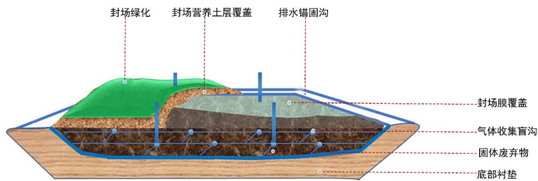
垂直防渗隔离示意图
