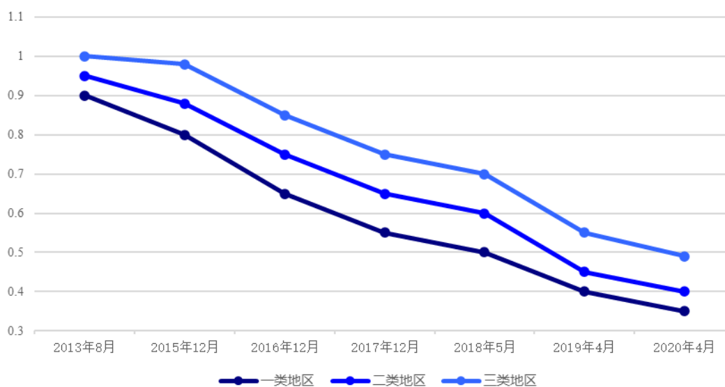
光伏发电标杆上网电价变动图（元/kWh，含税）
