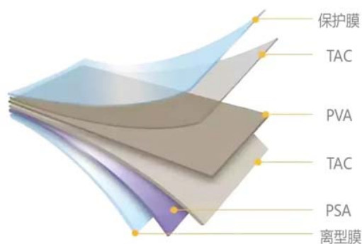
偏光片的构成
