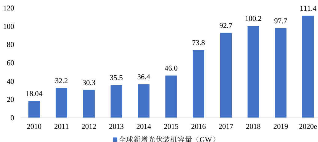
2010年-2019年全球新增光伏容量变化趋势
