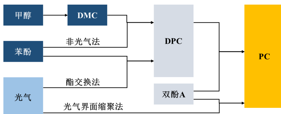
聚碳酸酯工艺路线简图
