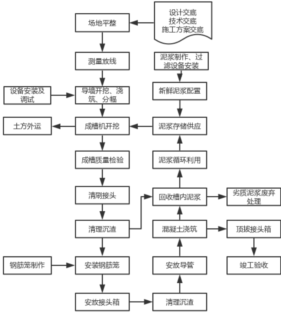
地下连续墙施工工艺流程图：
