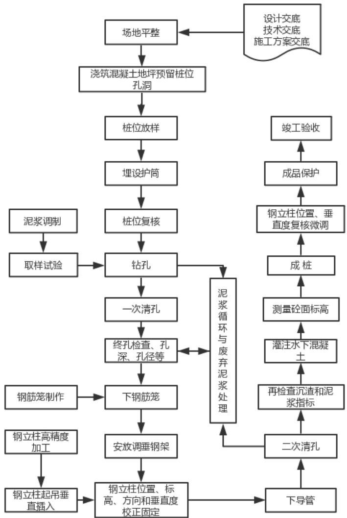
逆作法桩基施工工艺流程图：
