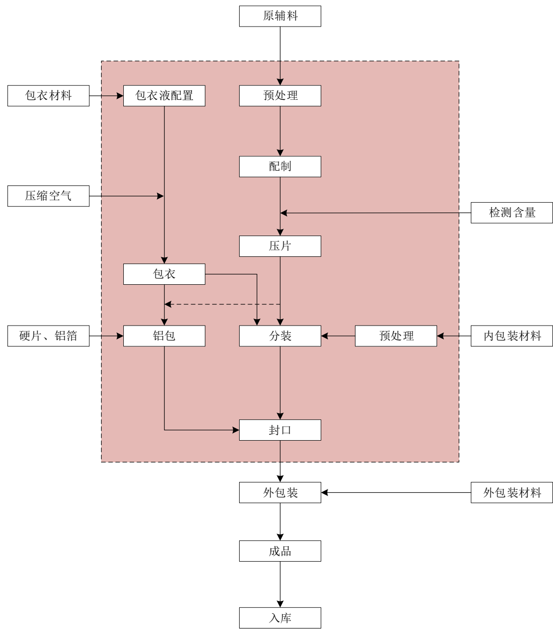
（4）片剂生产工艺流程图
