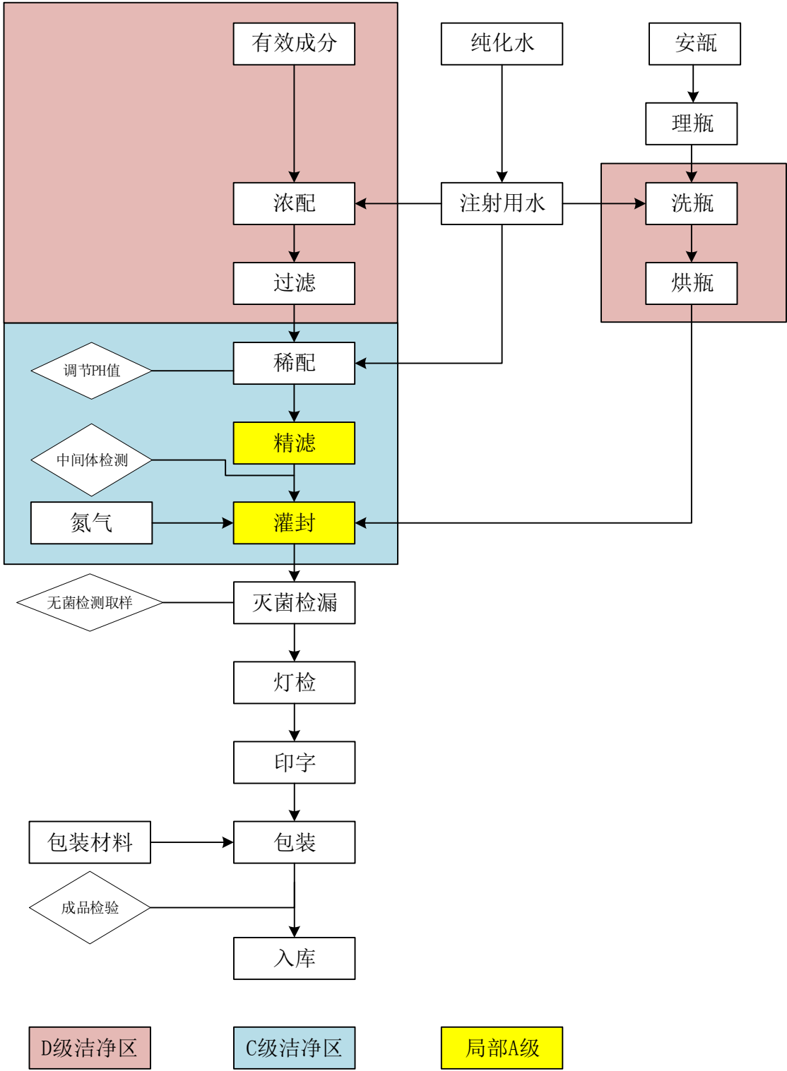
(5) 小容量注射剂生产工艺流程图
