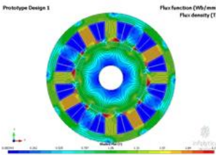
EPS电机磁场分析
