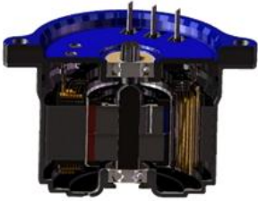
EPS电机产品剖面图
