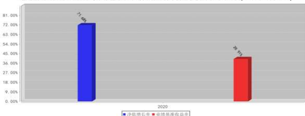
泰达宏利消费混合C基金每年净值增长率与同期业绩比较基准收益率的对比图(2020年12月31日)
