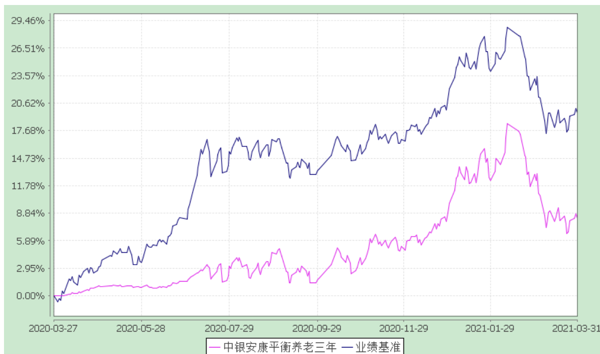
中银安康平衡养老目标三年持有期混合型发起式基金中基金（FOF） 份额累计净值增长率与业绩比较基准收益率历史走势对比图 （2020 年 3 月 27 日至 2021 年 3 月 31 日）
