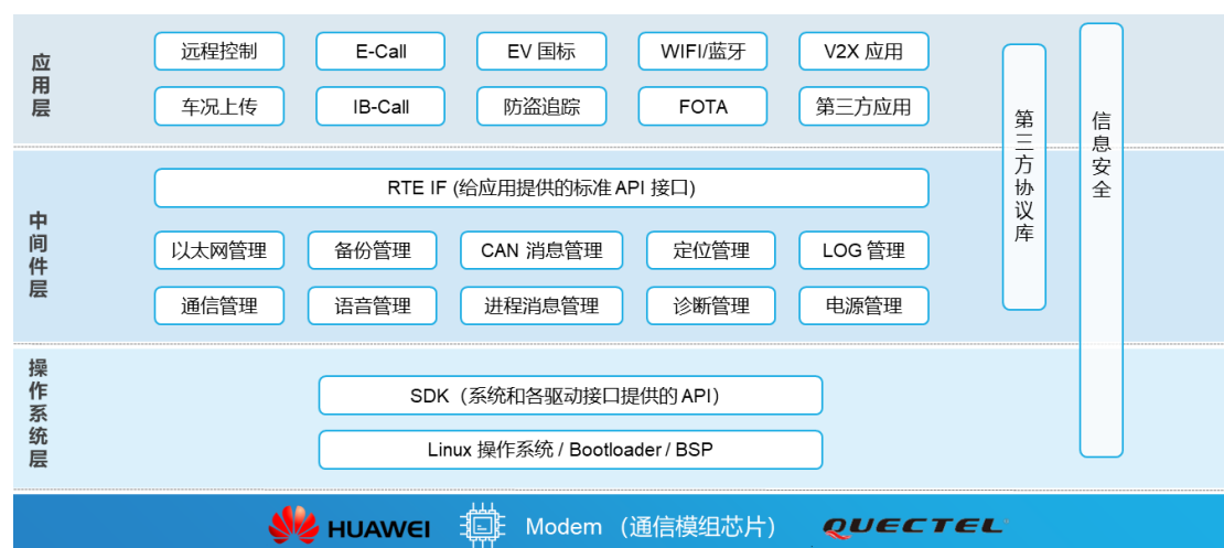
系统软件框架图
