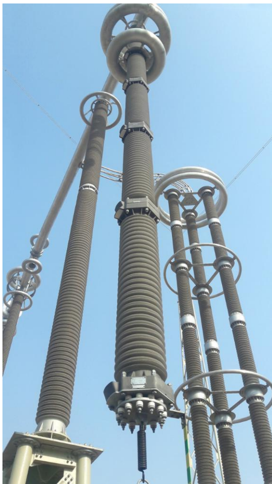
\pm 800\text{kV} 沂南换流站
