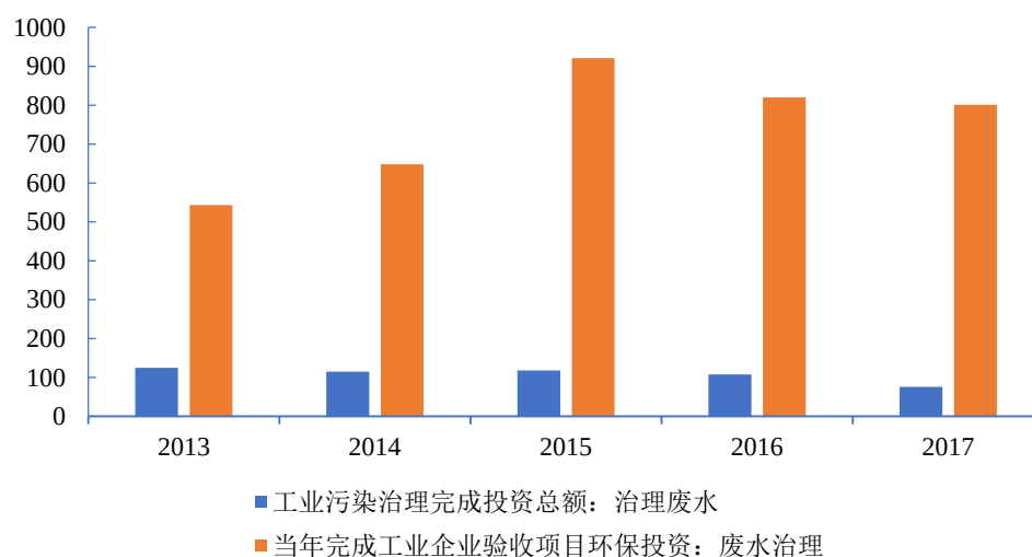
2013-2017年我国工业废水治理投资情况（亿元）
