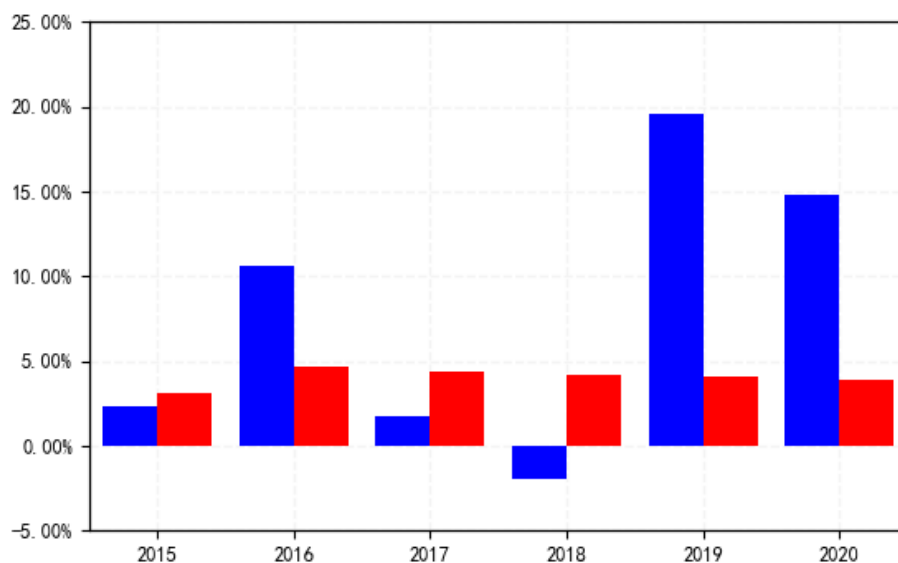
南方利众A类每年净值增长率与同期业绩比较基准收益率的对比图（2020年12月31日）
