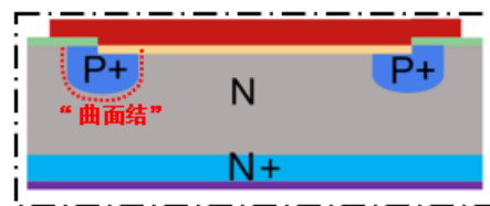
平面工艺下的芯片结构
