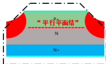
台面工艺下的芯片结构
