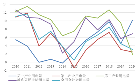
图 2：近年来中国分产业电力消费增速（%）
