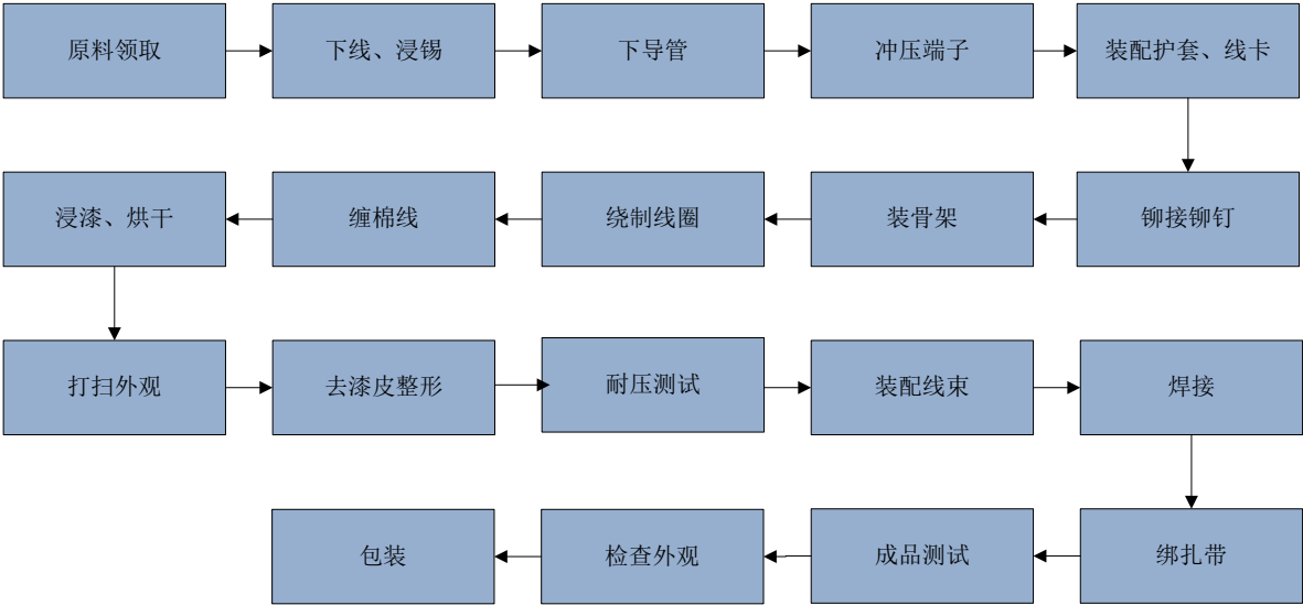
4、变流器生产流程图
