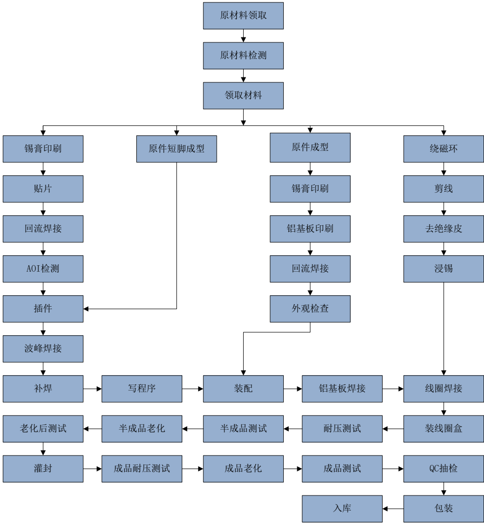
5、调压器/控制器生产流程图
