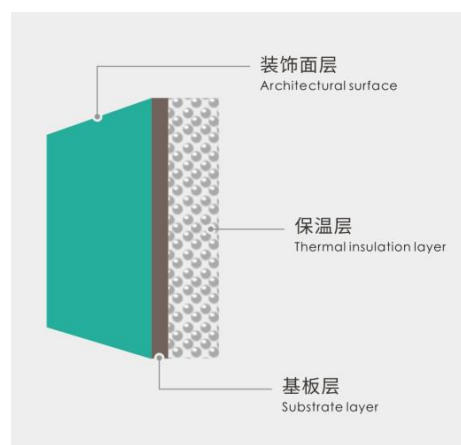
天工石产品构造示意图
