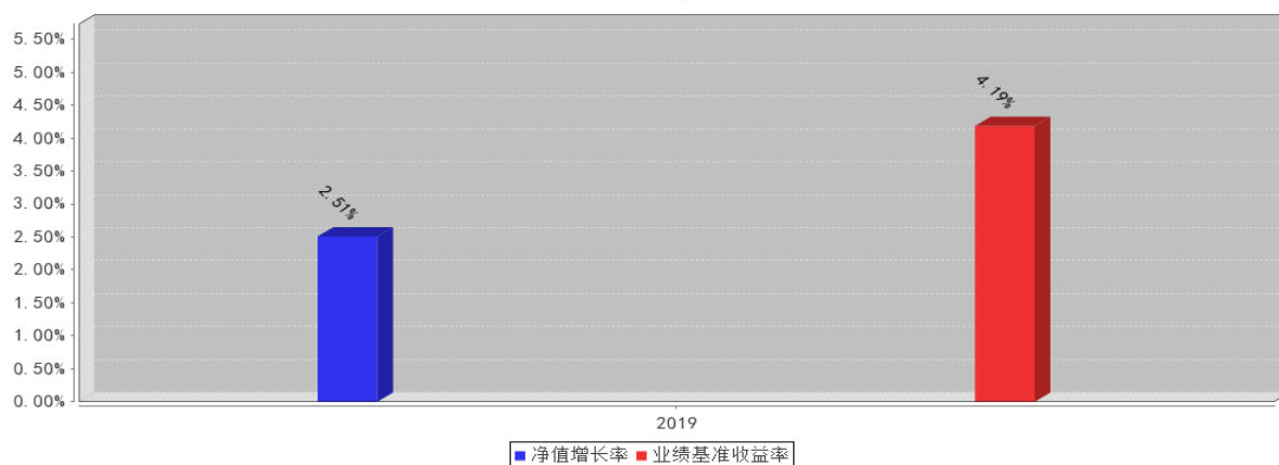
民生加银持续成长混合A基金每年净值增长率与同期业绩比较基准收益率的对比图(2019年12月31日)
