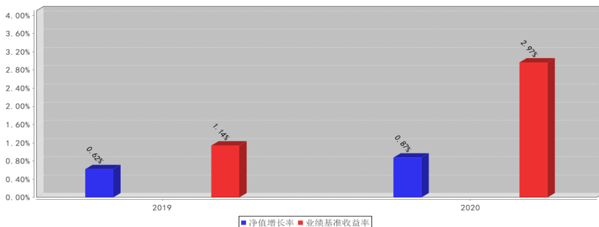
浦银安盛普丰纯债债券C基金每年净值增长率与同期业绩比较基准收益率的对比图(2020年12月31日)
