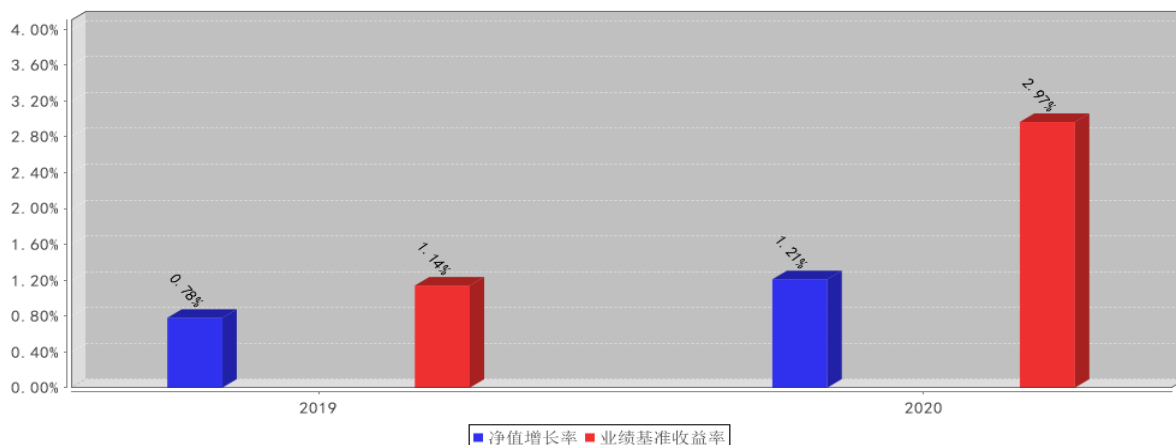
浦银安盛普丰纯债债券A基金每年净值增长率与同期业绩比较基准收益率的对比图(2020年12月31日)
