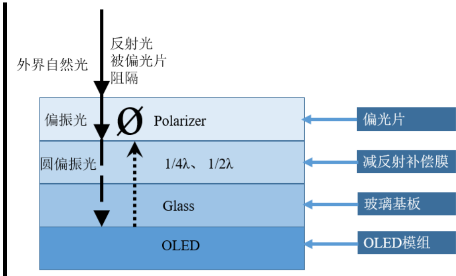
OLED 偏光片减反射位相差膜作用机理
