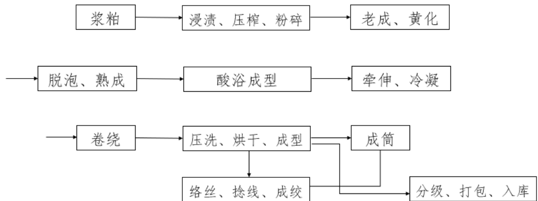
粘纤长丝生产工艺流程图
