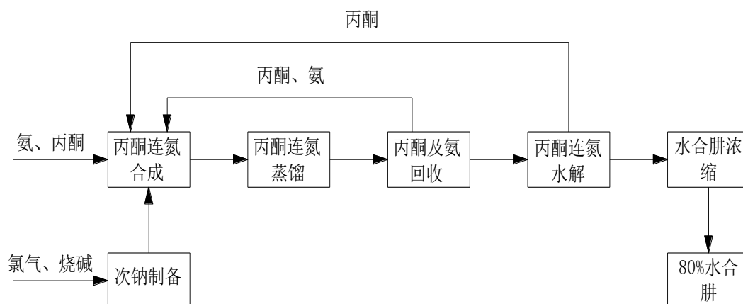
图：酮连氮法制 80% 水合肼工艺
