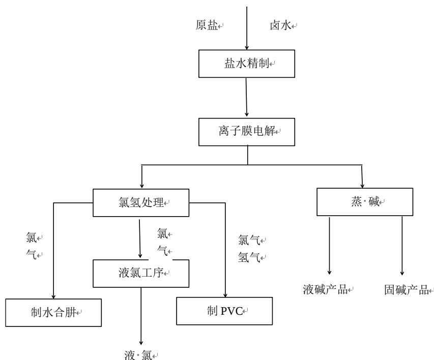
图：离子膜法制烧碱工艺
