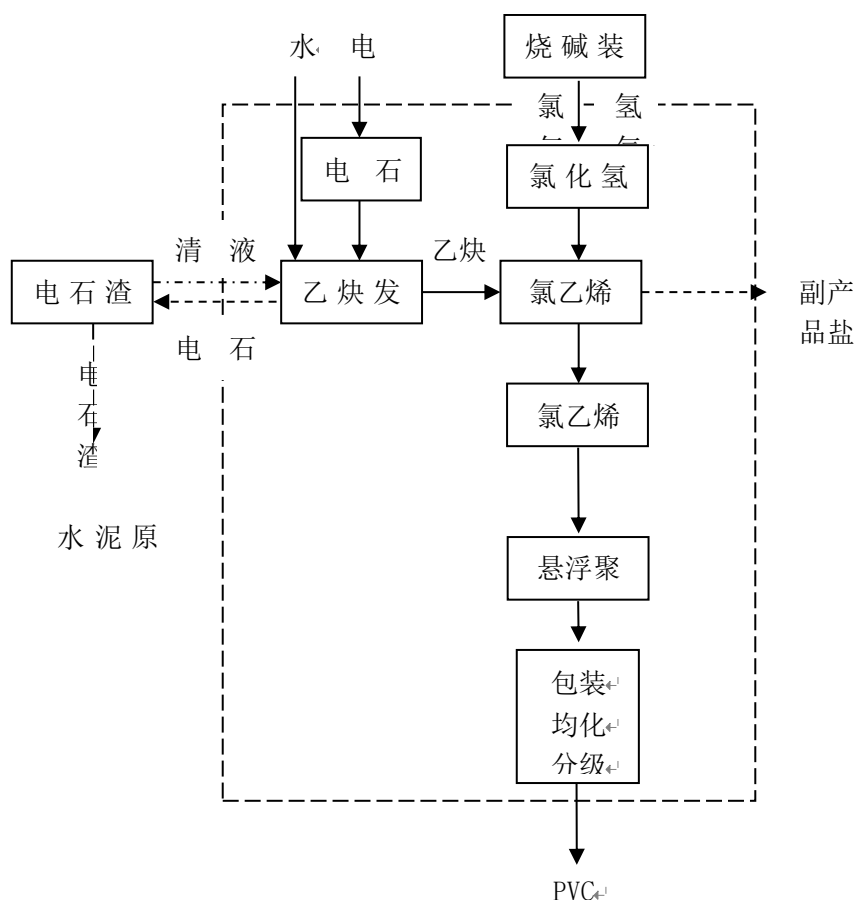
图：电石乙炔法
