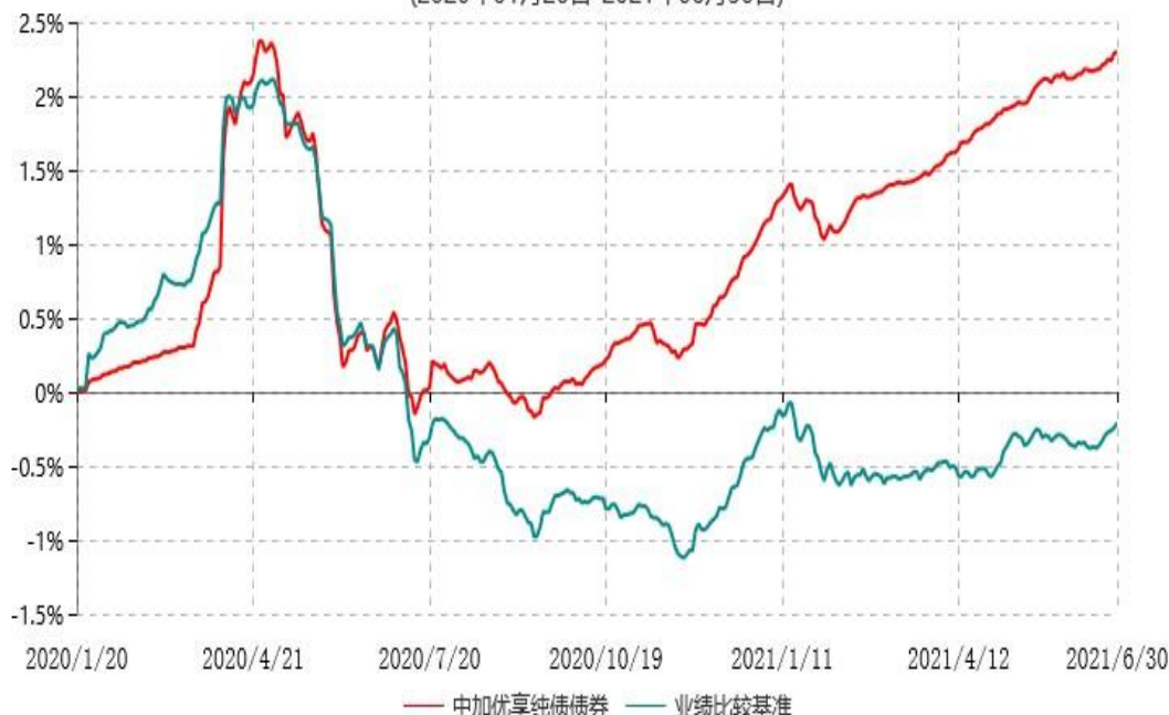
中加优享纯债债券型证券投资基金累计净值增长率与业绩比较基准收益率历史走势对比图 (2020年01月20日-2021年06月30日)
