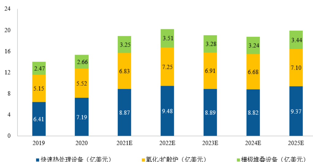
图表 9 全球热处理设备市场规模
