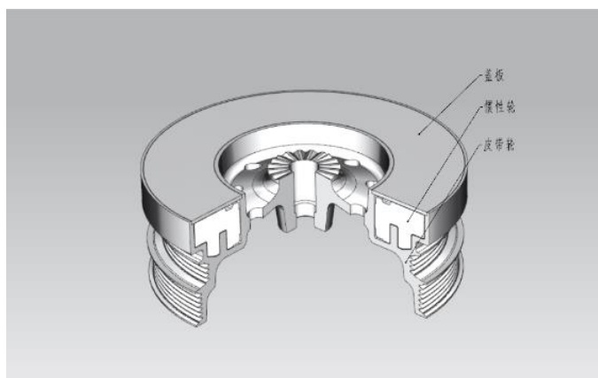
硅油减振器图解
