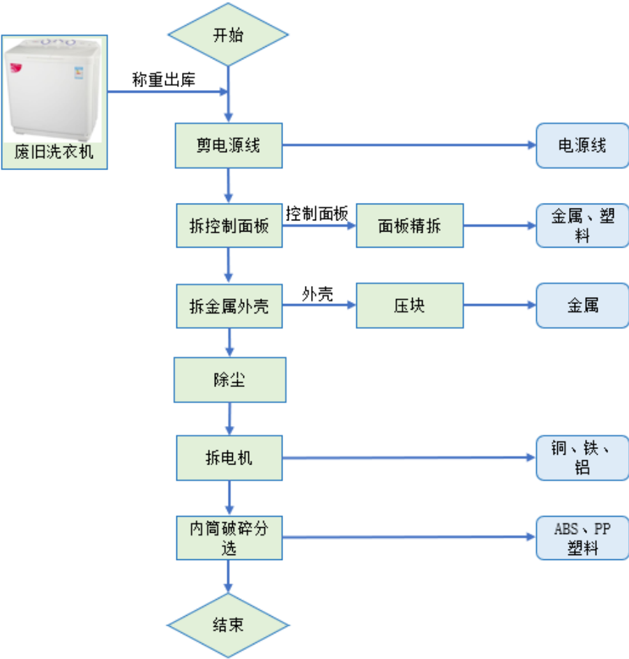
(4) 废旧洗衣机拆解工艺流程图
