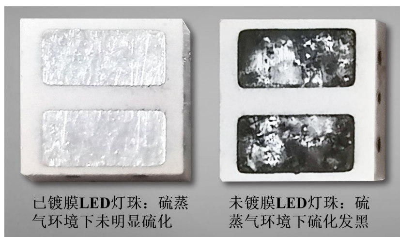
双层防液防气纳米薄膜：LED灯珠防硫化效果实物图
