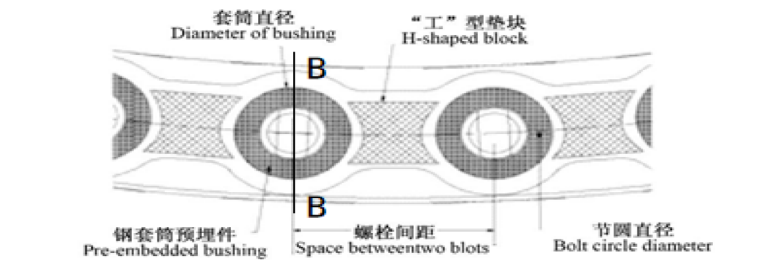
图 3：“预埋螺套” 连接细节图
