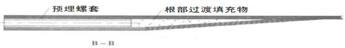
图 3：“预埋螺套” 连接细节图
