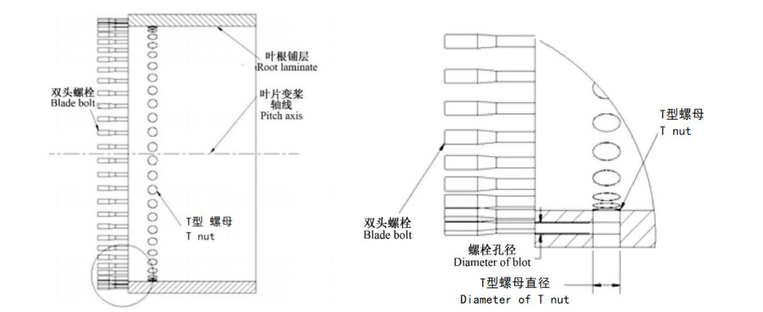
图 1：“T 型螺母” 连接方式示意图图 2：“T 型螺母” 连接细节图
