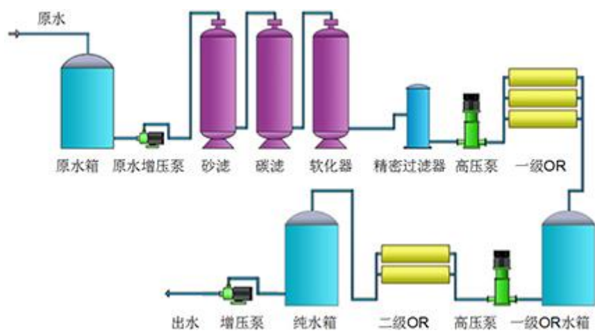
纯水处理示意图
