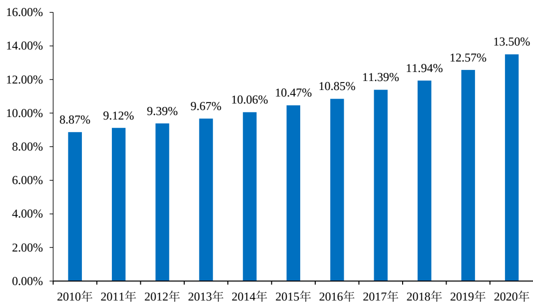
2010 年-2020 年我国 65 岁及以上人口占比
