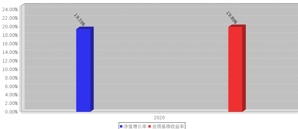
海通核心优势B基金每年净值增长率与同期业绩比较基准收益率的对比图(2020年12月31日)
