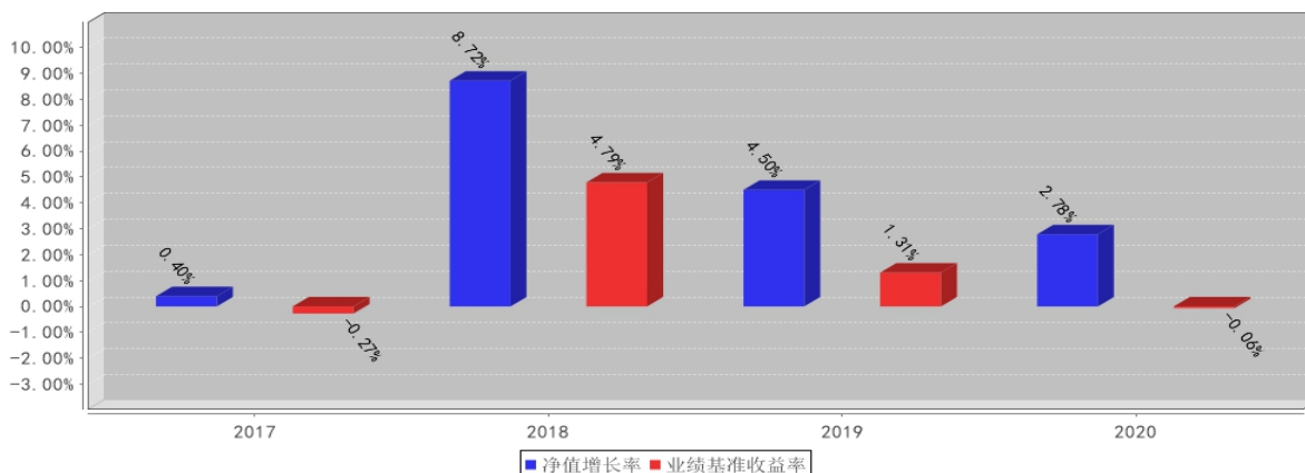
国寿安保安裕纯债半年定期开放债券发起式基金每年净值增长率与同期业绩比较基准收益率的对比图 (2020年12月31日)
