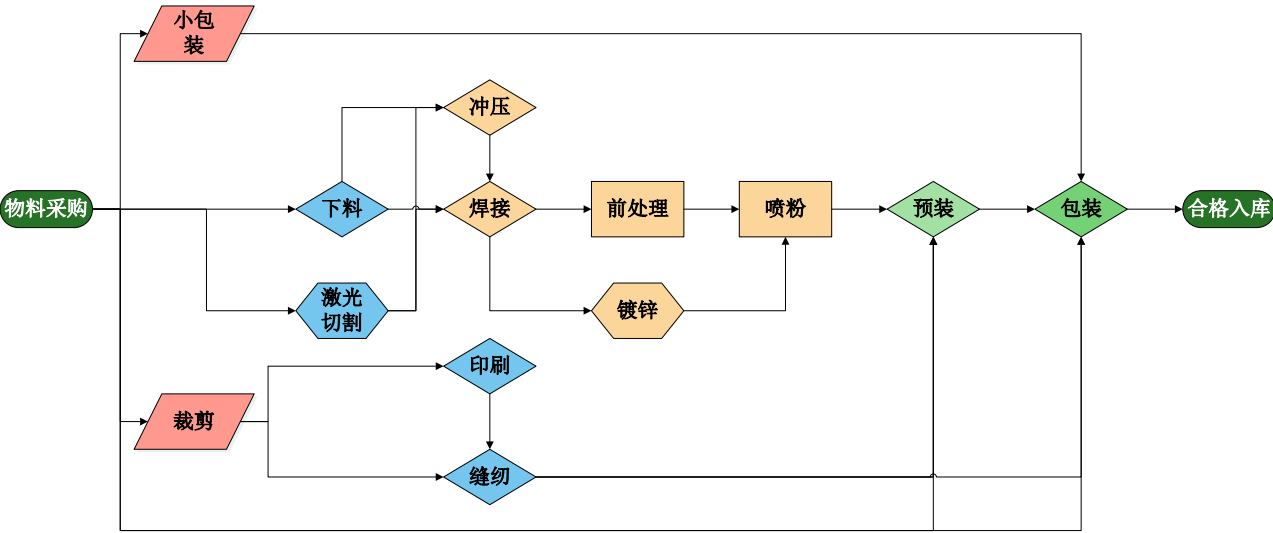
(2) 足球门、回球器及其他产品生产工艺流程图
