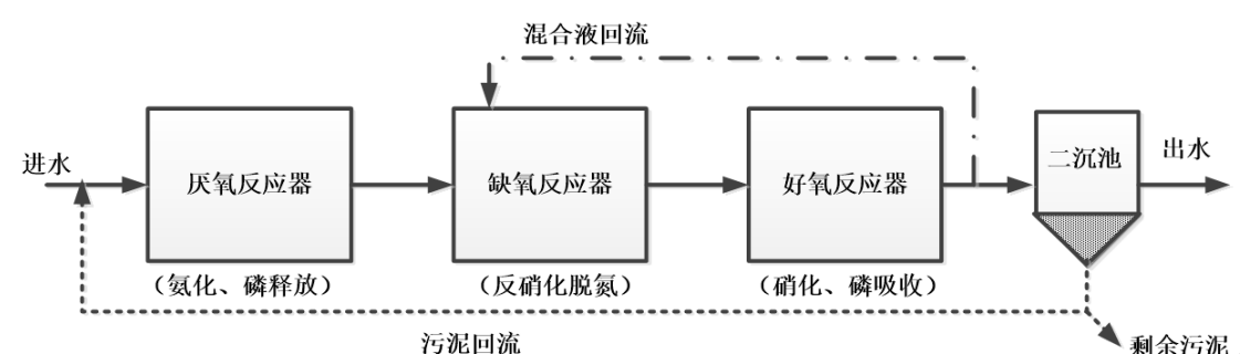
传统活性污泥法示意图（以“厌氧-缺氧-好氧”工艺为例）
