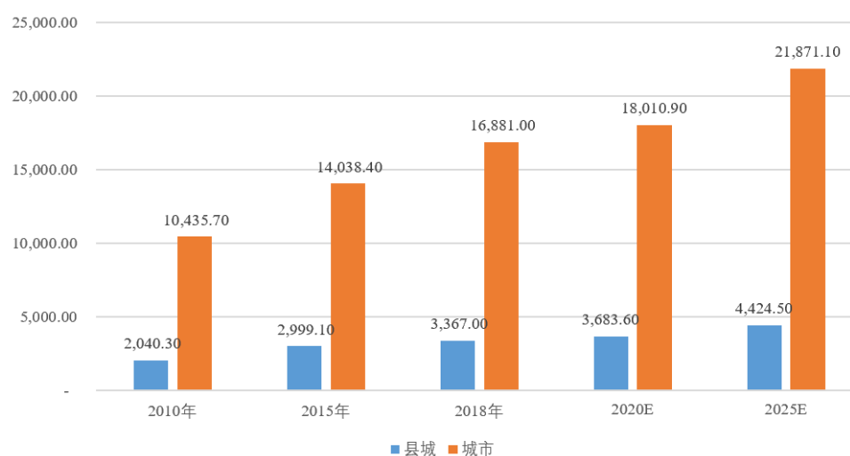
全国城镇污水处理厂处置能力预测（万立方米/日）
