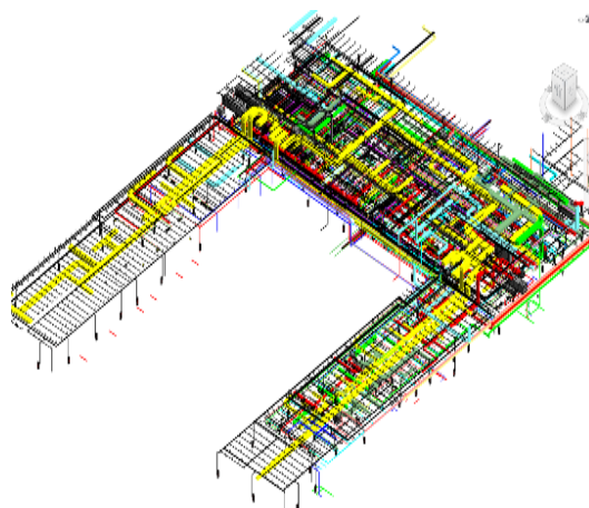
BIM 管线模型
