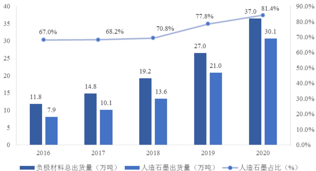
2016-2020年中国锂电池负极材料和人造石墨负极出货量情况
