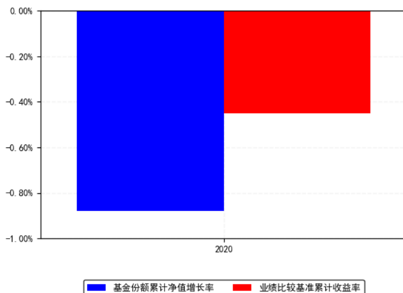
南方乐元中短利率债C每年净值增长率与同期业绩比较基准收益率的对比图（2020年12月31日）
