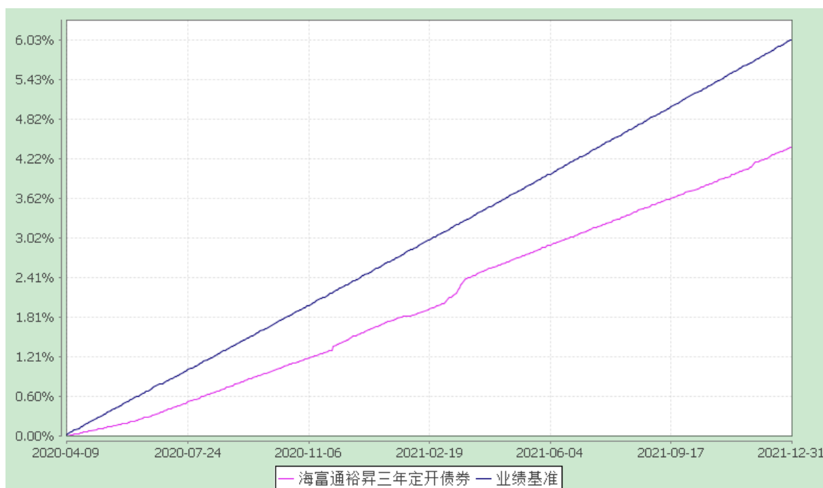
海富通裕昇三年定期开放债券型证券投资基金 份额累计净值增长率与业绩比较基准收益率历史走势对比图 (2020年4月9日至2021年12月31日)
