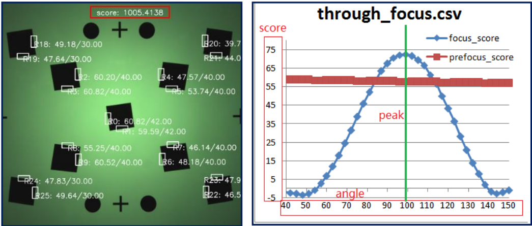
基于镜头光学特性的快速调焦算法示意图
