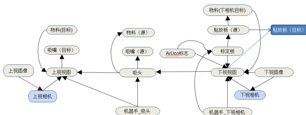
典型的自动贴装设备坐标及标定模型算法图
