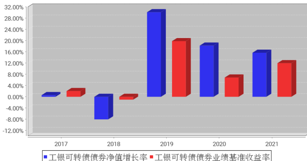
工银可转债债券基金每年净值增长率与同期业绩比较基准收益率的对比图
