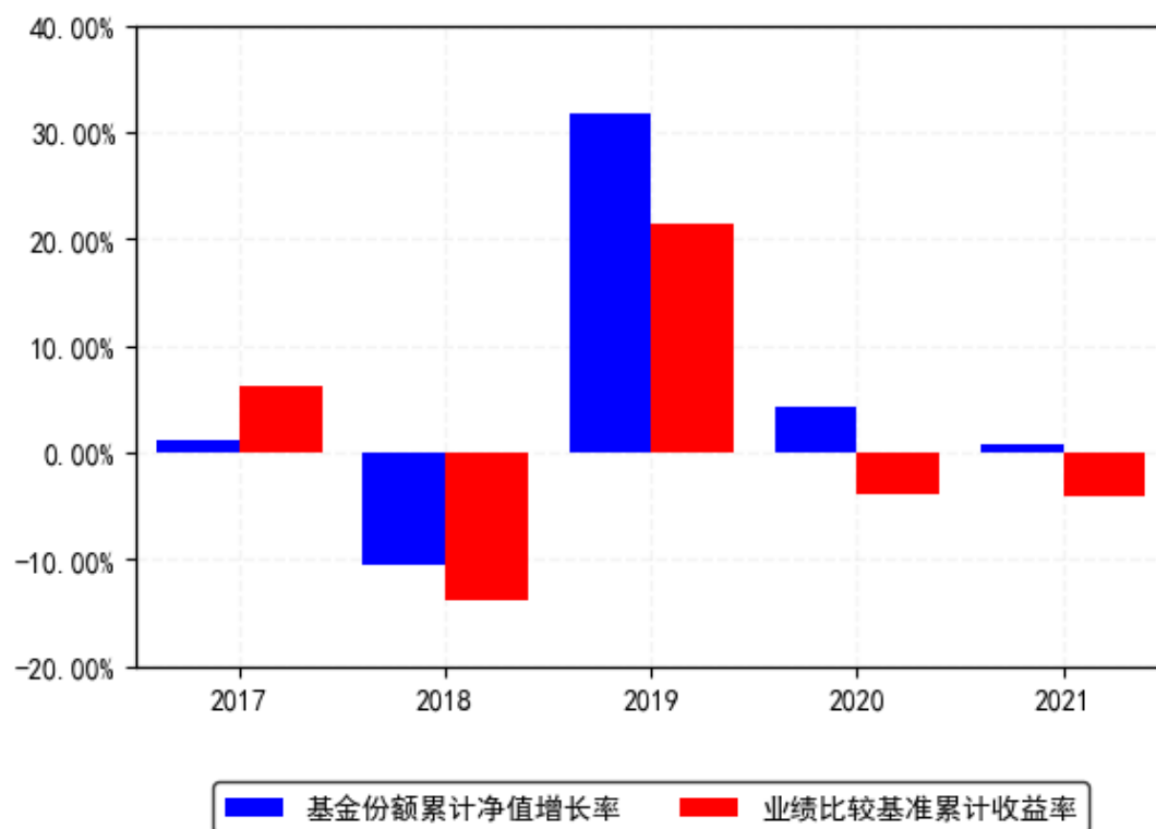
南方银行联接C每年净值增长率与同期业绩比较基准收益率的对比图
