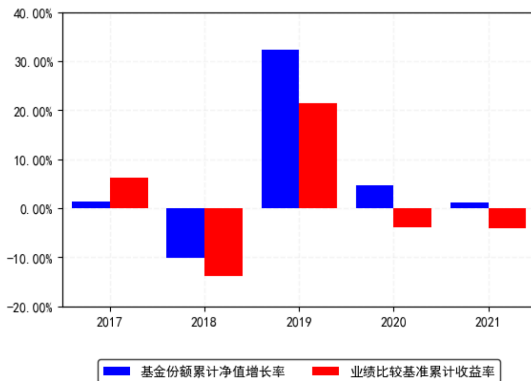
南方银行联接A每年净值增长率与同期业绩比较基准收益率的对比图
